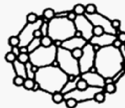
C_{36}
