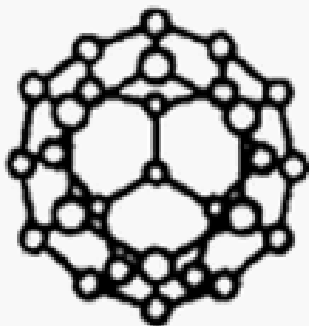
C_{28}
